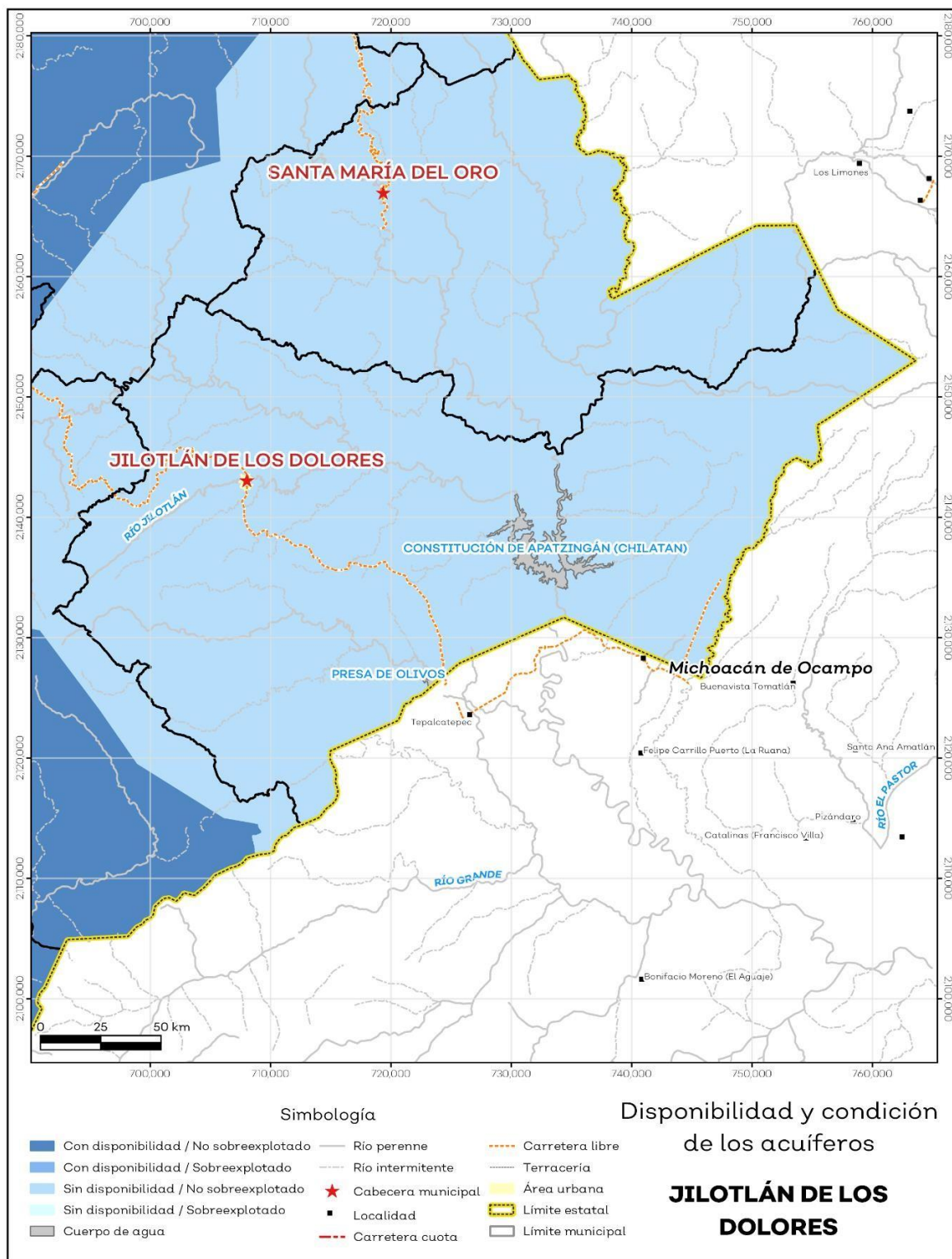
Mapa 6. Acuíferos
