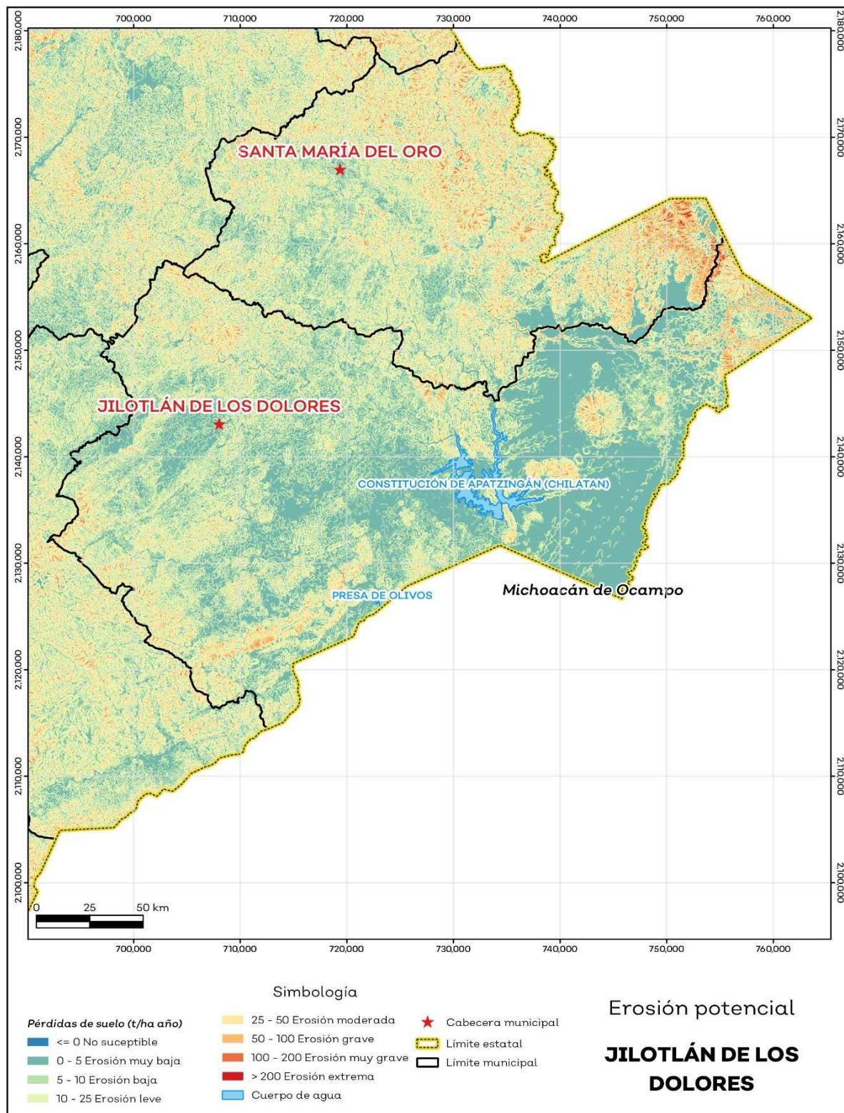
Mapa 8. Erosión potencial
